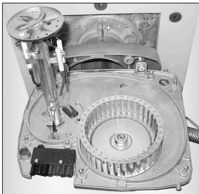
Рис. 11: Положение при обслуживании Logatop GE1H
