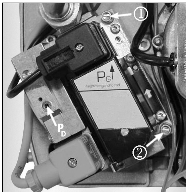
Рис. 9 Мультиблок Logatop GE1H Описание: ① Замер P G ② Замер P vor
