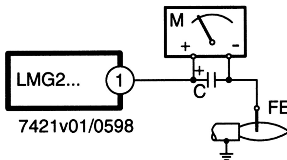
Рис. 13: Схема подключения измерительного прибора C Конденсатор электролитный 100...170 \mu F ; DC 10...25 V; для цифровых измерителей FE Электрод ионизации M Измеритель R_i max. 5000 \Omega
