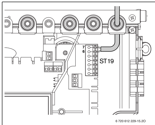
Рис. 18 Подключение регулятора
