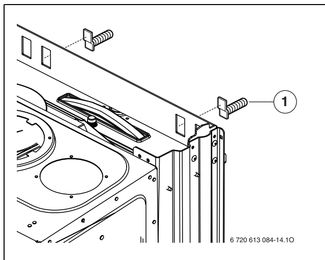
Рис. 9 Подвешивание прибора
